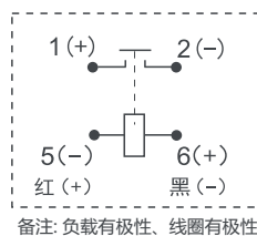
接线图 Wiring diagram
