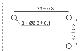
安装孔尺寸 Mounting hole size
